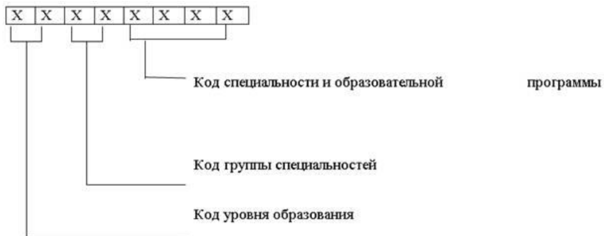
Рисунок 1 - Структура кодирования
